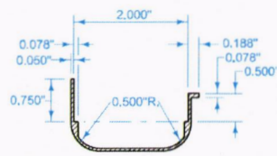
EDGE MOLDING
